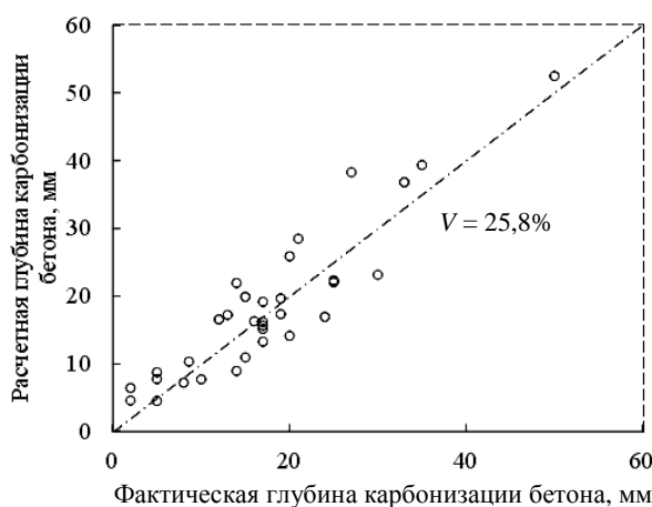
Рисунок 2. – Соотношение фактических и расчетных значений карбонизации бетона мостовых железобетонных конструкций
