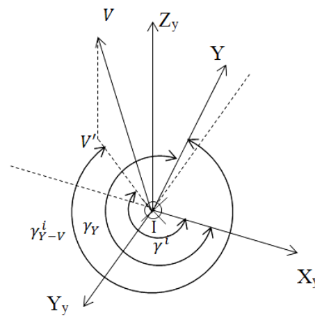
V – визирная ось тахеометра; V' – проекция визирной оси на плоскость X_y Y_y ; Y – ось Y в принятой нами системе координат; \gamma^i – горизонтальный угол между осью X_y и проекцией визирной оси тахеометра на плоскость X_y Y_y ; \gamma_Y – горизонтальный угол между осью X_y и осью Y ; \gamma_{Y-v^i} – горизонтальный угол между осью Y и проекцией визирной оси тахеометра на плоскость X_y Y_y в момент фотографирования для снимка i
