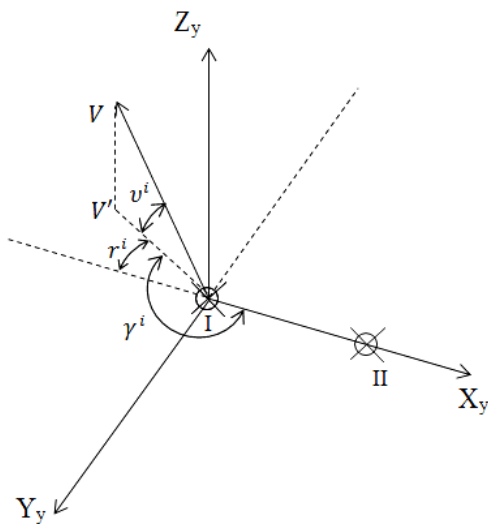
V – визирная ось тахеометра; V' – проекция визирной оси на плоскость X_y Y_y ; v^i – вертикальный угол между осью V и её проекцией V' для снимка с номером i ; \gamma^i – горизонтальный угол между проекцией визирной оси V' и осью X_y для снимка с номером i ; r – румб угла \gamma
