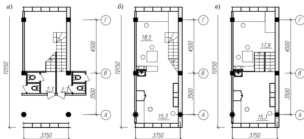
Рис. 3. Жилые ячейки типа F и 2F в доме Наркомфина по проекту М. Гинзбурга, М. Милиниса и инженера С. Прохорова в Москве: а – средний уровень, ячейки типа F и 2F; б – нижний уровень, ячейка типа F; в – верхний уровень, ячейка типа 2F
