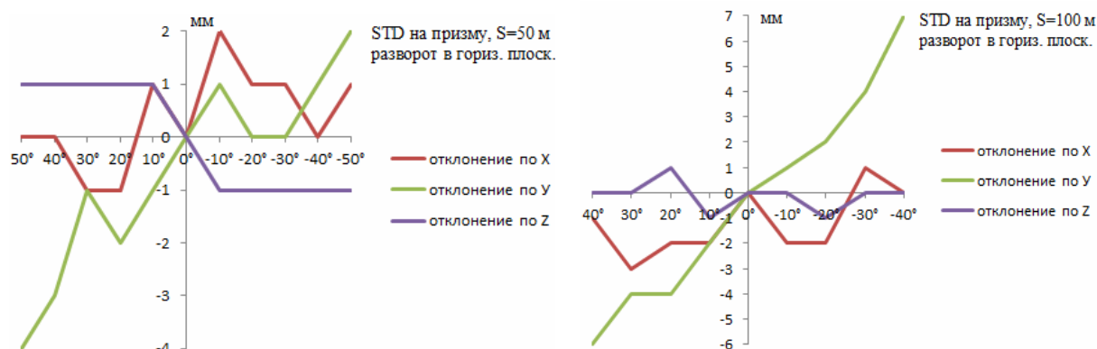
Рисунок 2 – Зависимость погрешности измерения направлений и линий от угла разворота призмного отражателя в горизонтальной плоскости
