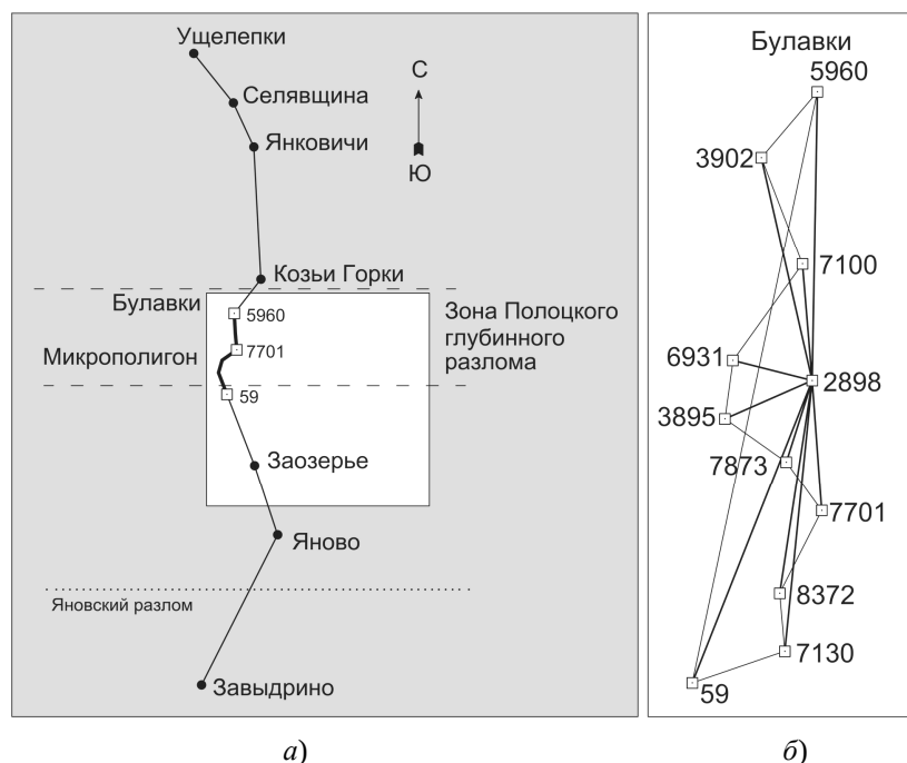
Рис. 1. Схема инструментальных исследований в Полоцко-Курземском поясе тектонических разломов:
