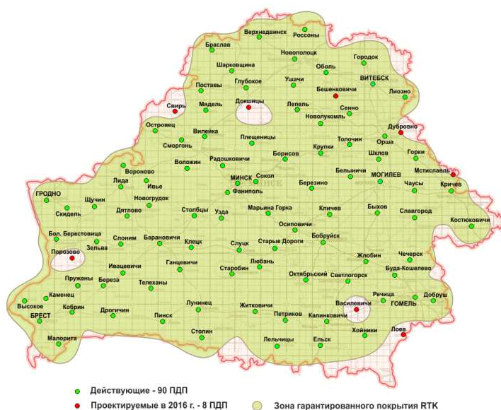
Рисунок 1 – Схема расположения ПДП
