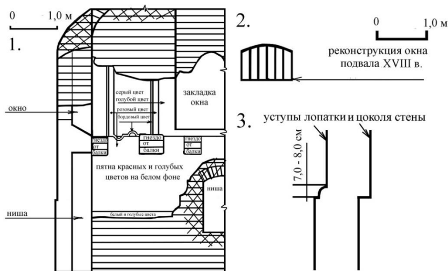
1. – общий план; 2. – окно подвала южной стены; 3. – профиля выступа между стеной и цоколем на уровне лопатки и прясла
