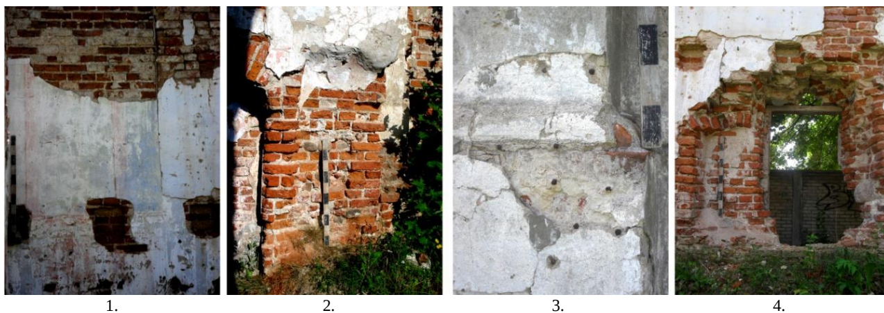
1. – южная стена апсиды: видны остатки росписи, часть закладки окна и пробитые гнёзда под балки перекрытия XX в.; 2. – растёс западного откоса большой арки для устройства диаконских дверей; 3. – восточный фасад: низ лопатки с гвоздями для укрепления штукатурки; 4. – южная стена: разбитая первоначальная ниша, видны пробитые гнёзда под балки перекрытия XX в.
