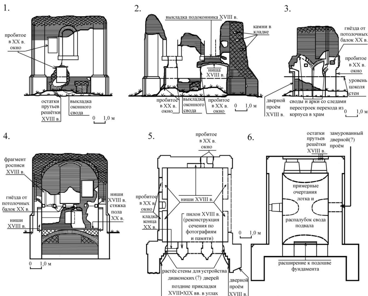
1. – фасад южной стены; 2. – фасад восточной стены; 3. – фрагмент фасада северо-западной части апсиды на стыке с южным выступом основной части храма (видны следы конструкций перехода между костёлом и корпусом); 4 – общий вид (разрез) южной стены апсиды со стороны интерьера подвала и верхнего помещения (с частичной реконструкцией); 5. – план верхнего помещения на уровне нижнего яруса с частичной реконструкцией; 6. – план подвала с частичной реконструкцией контуров свода
