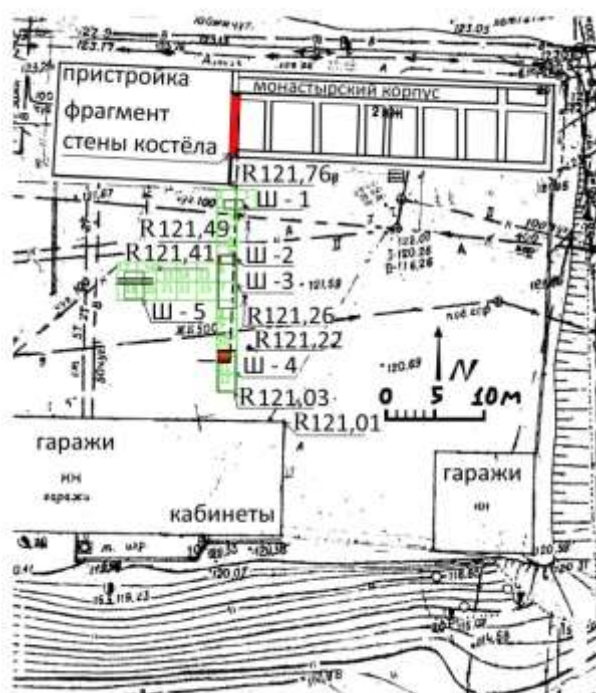
Рисунок 1. – План бывшего Францисканского монастыря с обозначением найденных фрагментов стен костёла (отмечены красным)
