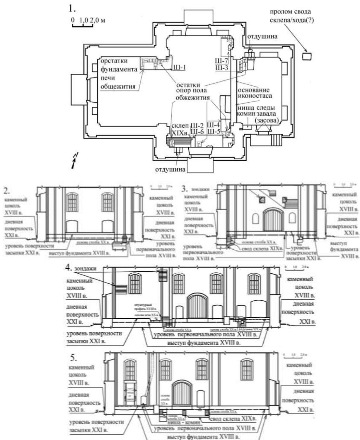
Рисунок 1. – План (1), поперечные (2, 3) и продольные (4, 5) разрезы храма св. Николая в с. Ропно
