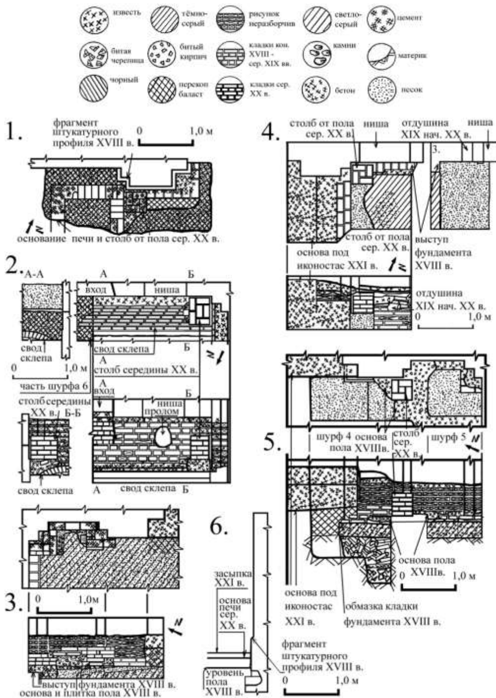
1. – шурф 1 у северо-западной подкупольной опоры; 2. – шурф 2 с частью шурфа 6 со сводом южной стороны склепа; 3. – шурф 7 выкладка сер. XX в с плиткой пола и слоем черепицы; 4. – шурф 3 у основания иконостаса с отдушиной в стене; 5. – шурфы 4 и 5 с врезкой у фундамента; 6. – округлый профиль цоколя базы на северо-западной опоре
