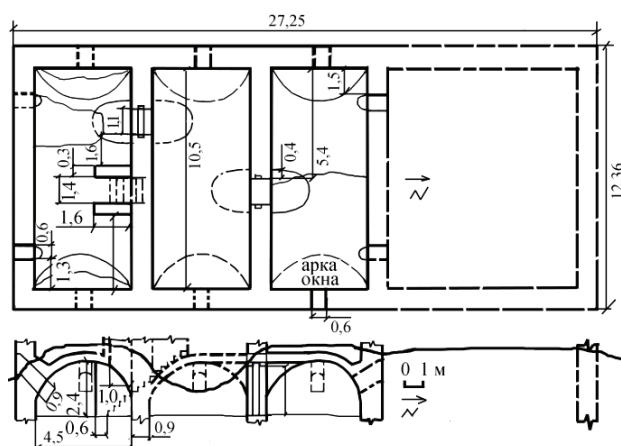
Рис. 6. План подвала панского дома с частичными обмерами и реконструкцией
