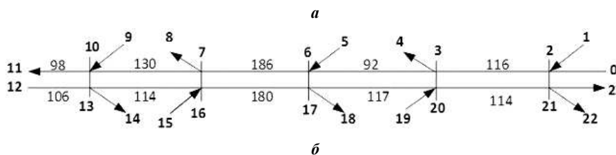
а – общий вид; б – представление в виде ориентированного графа; 0–11, 12–23 – основные направления транспортных потоков
