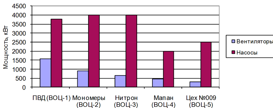
Рисунок 5. – Оценка потребления электроэнергии вентиляторами и насосами градирен производств Завода «Полимир» ОАО «Нафтан»
