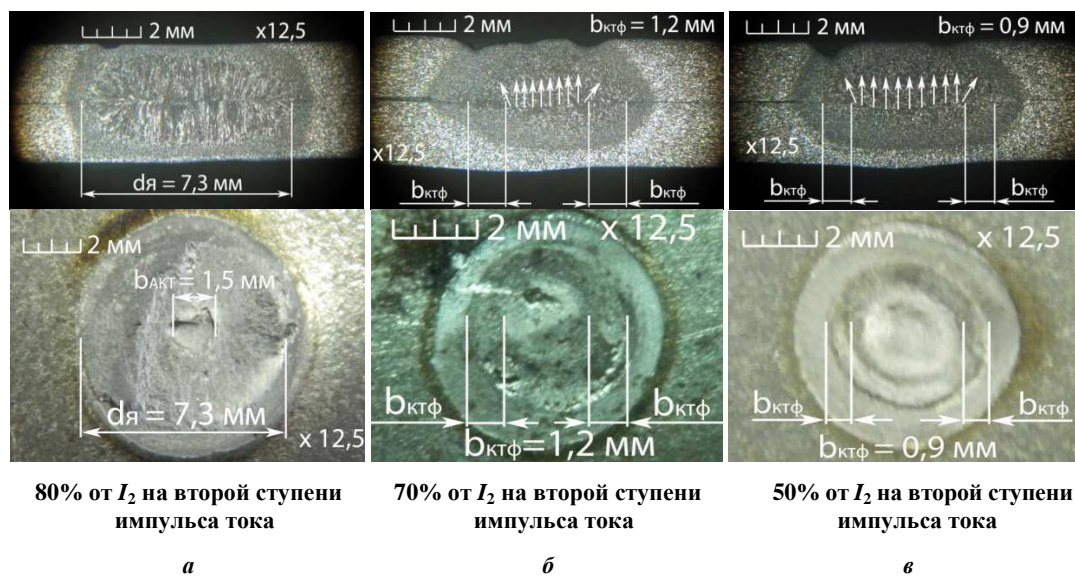
d_я – диаметр литого ядра; b_{акт} – зона активации; b_{ктф} – ширина кольца твердой фазы (стрелками показаны направления выдавливания металла при сварке)
