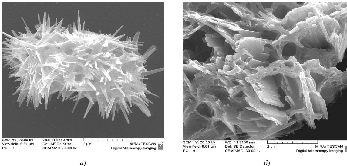
Рис. 5. Микроструктура дисперсной фазы kSulCa ПСМ до испытаний (а) и после (б)
