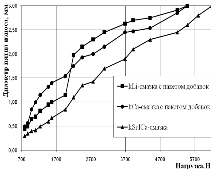
Рис. 6. Нагрузочные кривые пластичных смазок различного состава
