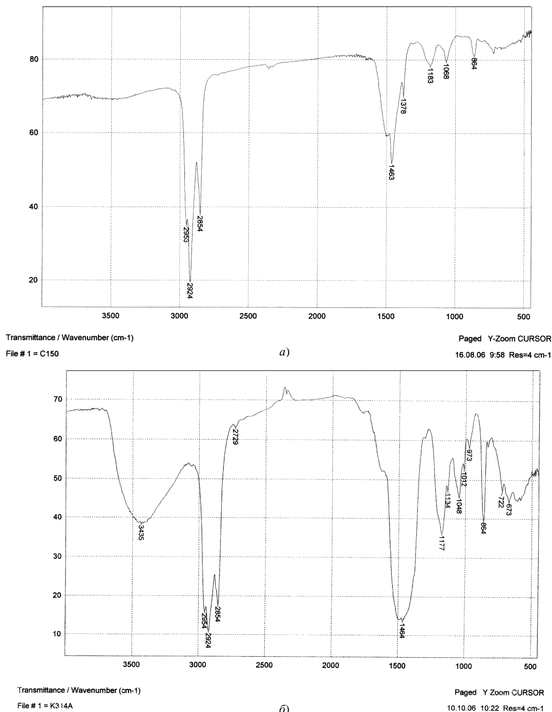
Рис. 1. ИК-спектры сульфатных присадок С-150 (а) и К-314 (б)
