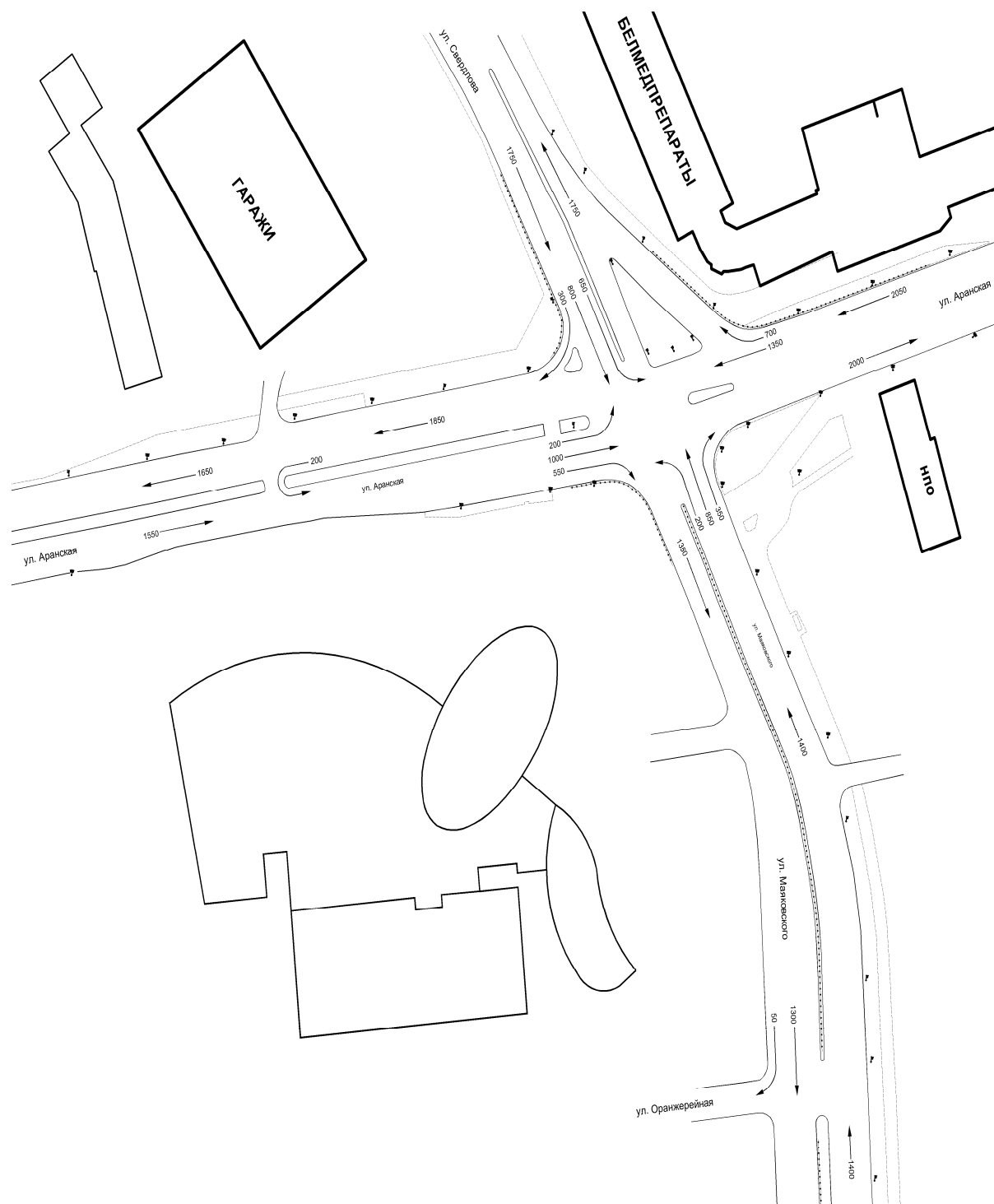
Рис. 4. Организация дорожного движения в исследуемом районе (вариант 1)
