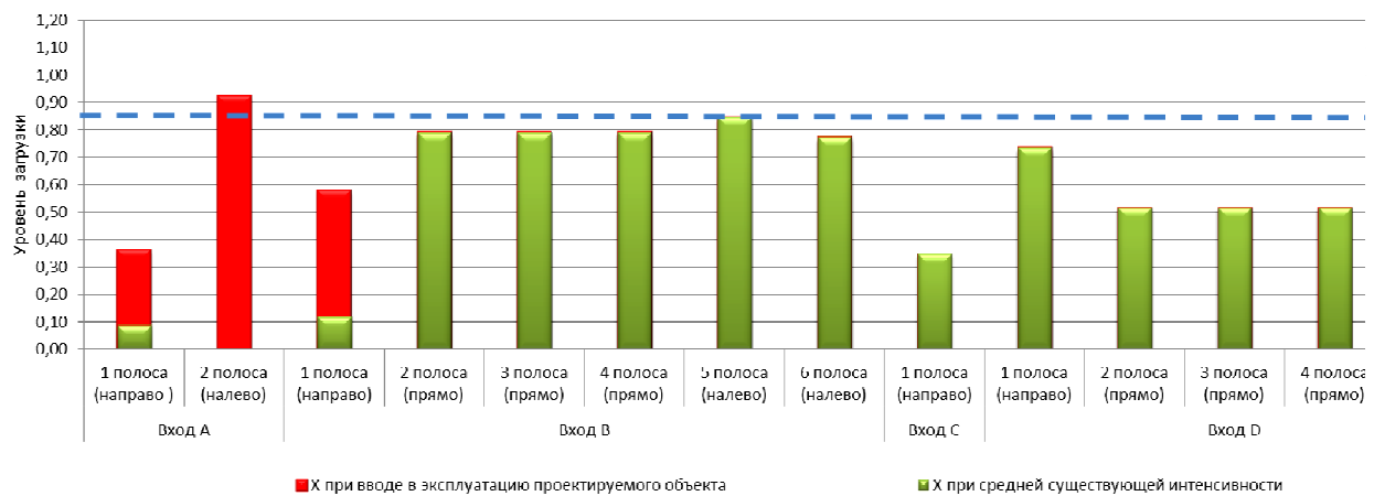
Рис. 9. Предполагаемый уровень загрузки на перекрестке улиц Маяковского и Оранжерейная (3 фазы, с улицы Оранжерейной во всех направлениях, разрешен левый поворот с улицы Маяковского на Оранжерейную)
