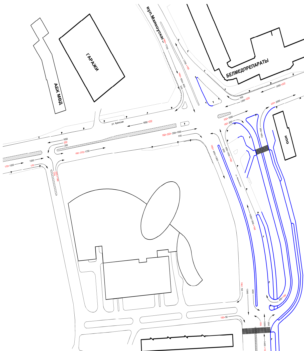
Рис. 5. Организация дорожного движения в исследуемом районе (вариант 2)
