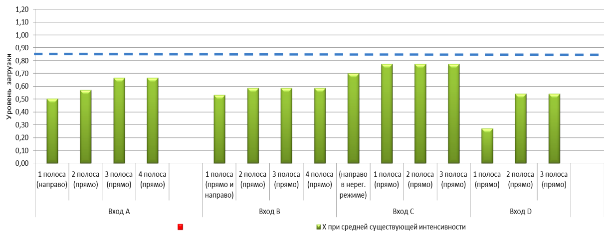
Рис. 2. Предполагаемый уровень загрузки на перекрестке улиц Аранская и Маяковского: а – схема организации дорожного движения с устройством левоповоротного съезда и сохранением левоповоротного движения с улицы Маяковского (в сторону ул. Могилевской). На перекрестке улиц Аранская и Маяковского применяется 3-хфазная схема регулирования; б – схема организации дорожного движения с устройством левоповоротного съезда и запрещением левоповоротного движения с улицы Маяковского (в сторону улицы Могилевской). На перекрестке улиц Аранская и Маяковского применяется 2-фазная схема регулирования
