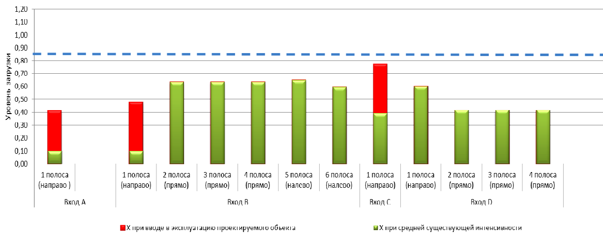
Рис. 7. Предполагаемый уровень загрузки на перекрестке улиц Маяковского и Оранжерейная (2 фазы с улицы Оранжерейной только направо; В – со стороны улицы Архангельской)
