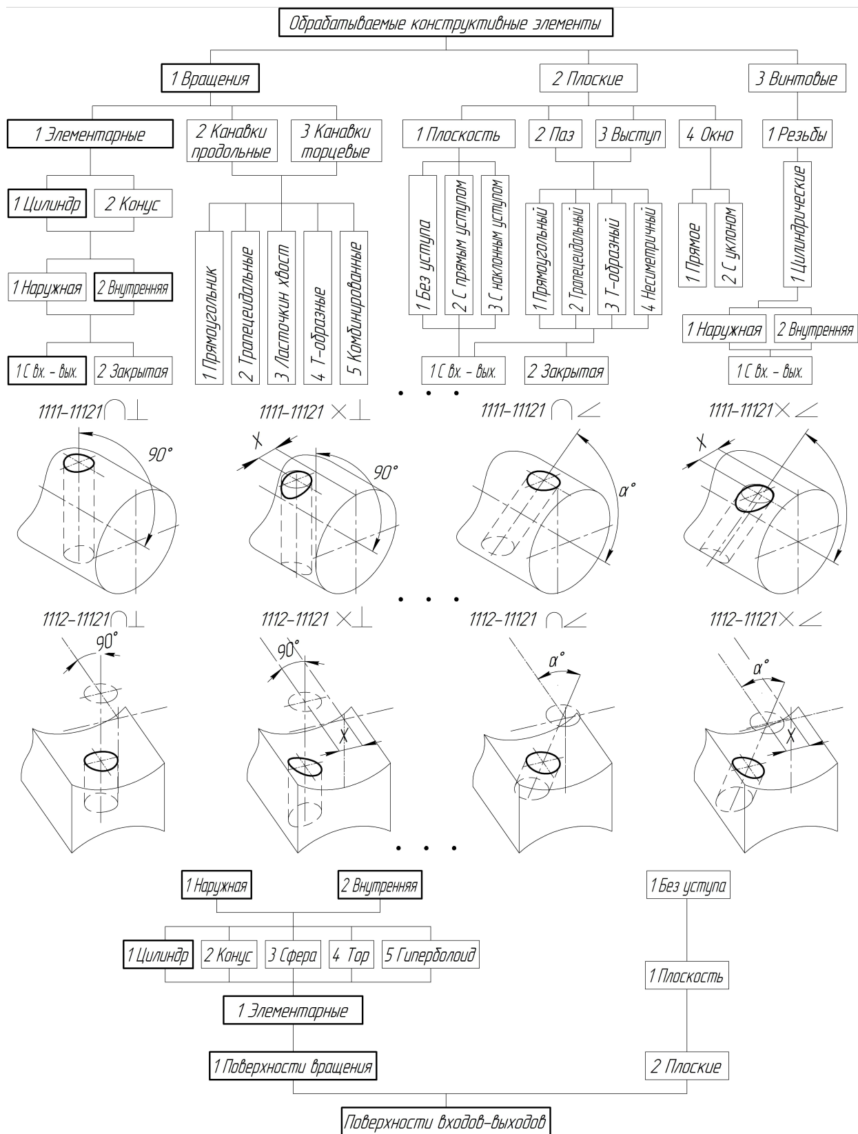
Рисунок 1. – Элементы системы классификации взаимных расположений обрабатываемых конструктивных элементов и поверхностей входов-выходов
