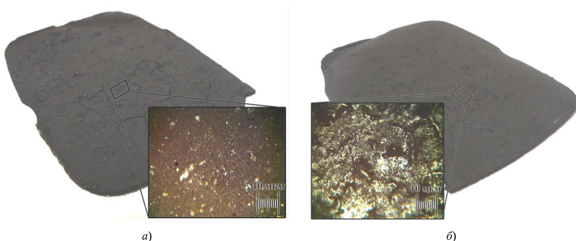
Рис. 1. Оптические микроснимки рабочей поверхности (а) и обратной стороны (б) образца № 2 (30 масс. % шунгита)
