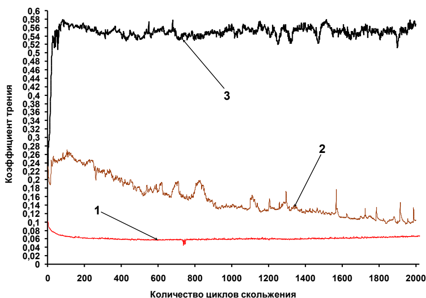
Рис. 3. Сравнительная диаграмма изменения коэффициента трения от длительности изнашивания (без смазки) поверхности стали У8 до и после ТГХО [6].
