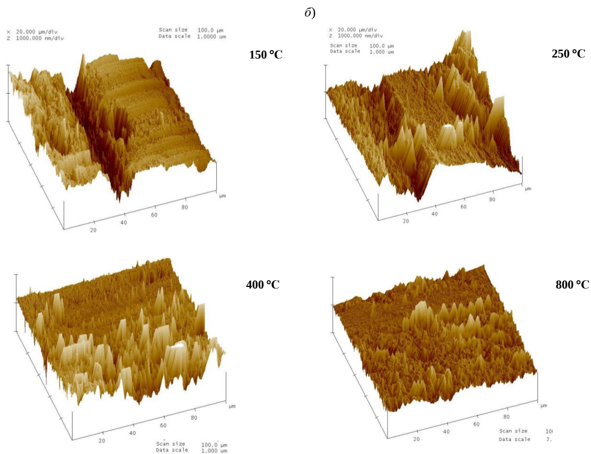
Рис. 4 – Окончание. Изменение морфологии поверхности стали У8 от температуры последующего нагрева (б)
