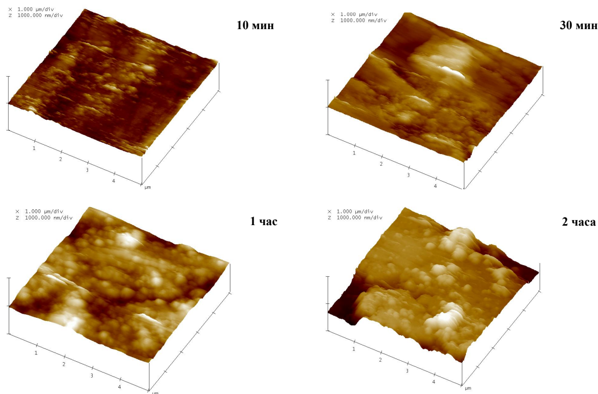
Рис. 4. Изменение морфологии поверхности стали У8 от времени гидрохимической обработки (a).
