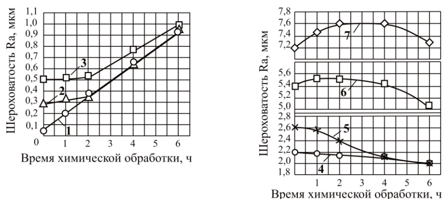
Рис. 5. Зависимость шероховатости поверхности стали У8 с покрытием от времени ГХО и качества исходной поверхности: 1 – 7 – номер образца (см. табл. 2)
