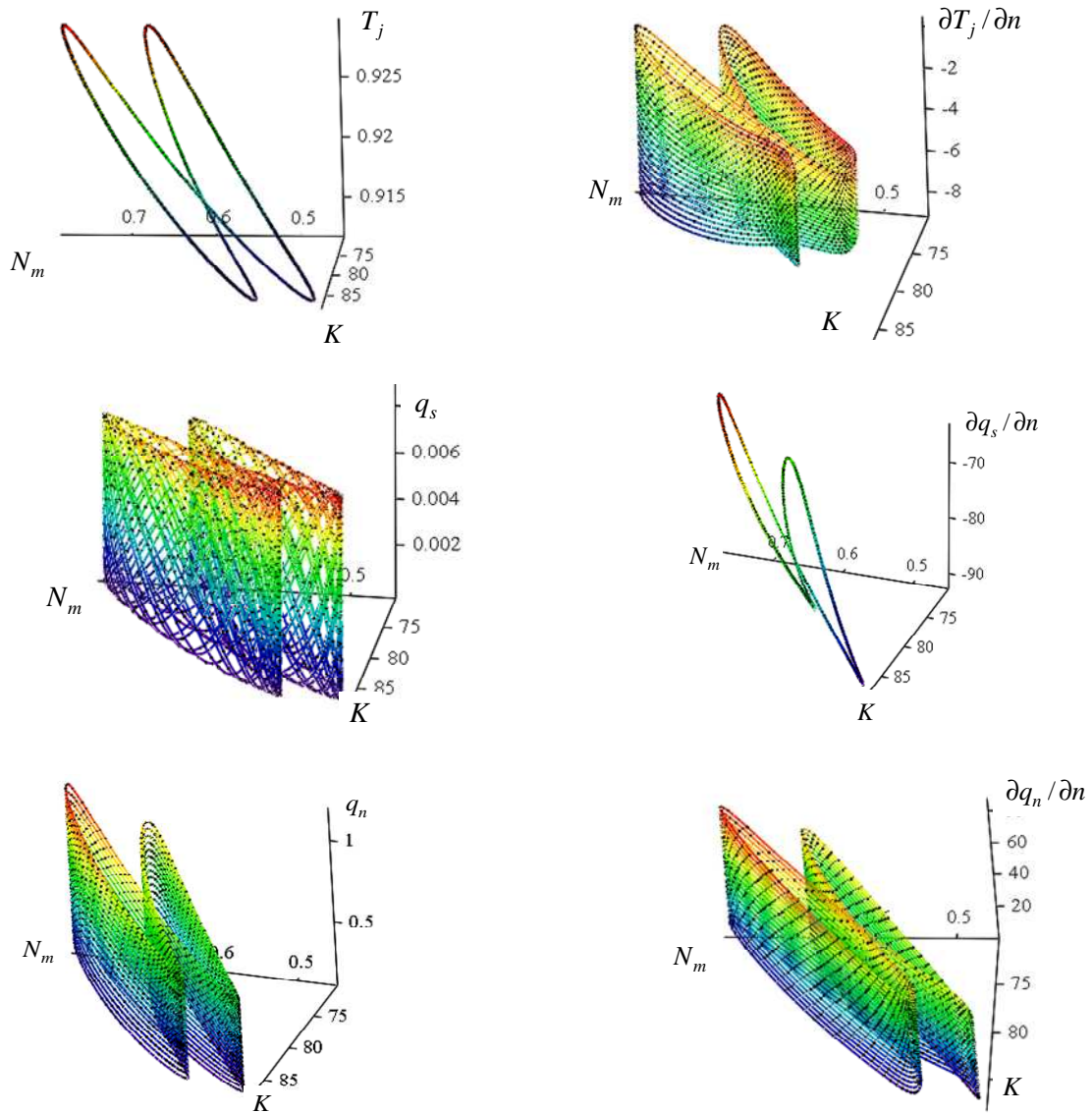
Рисунок 1. – Тепловое состояние дендрита в конечной окрестности его вершины для режима колебаний (15): n_1 = 1 ; a_1 = 0,1 ; \omega_1 = 0,5 ; a_2 = 0,4 ; \omega_2 = 1 ; q^1_* = 0,01 , y = 0,01
