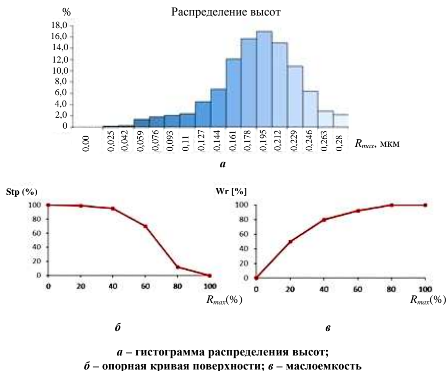
Рисунок 8. – Топографические характеристики поверхности после MAO
