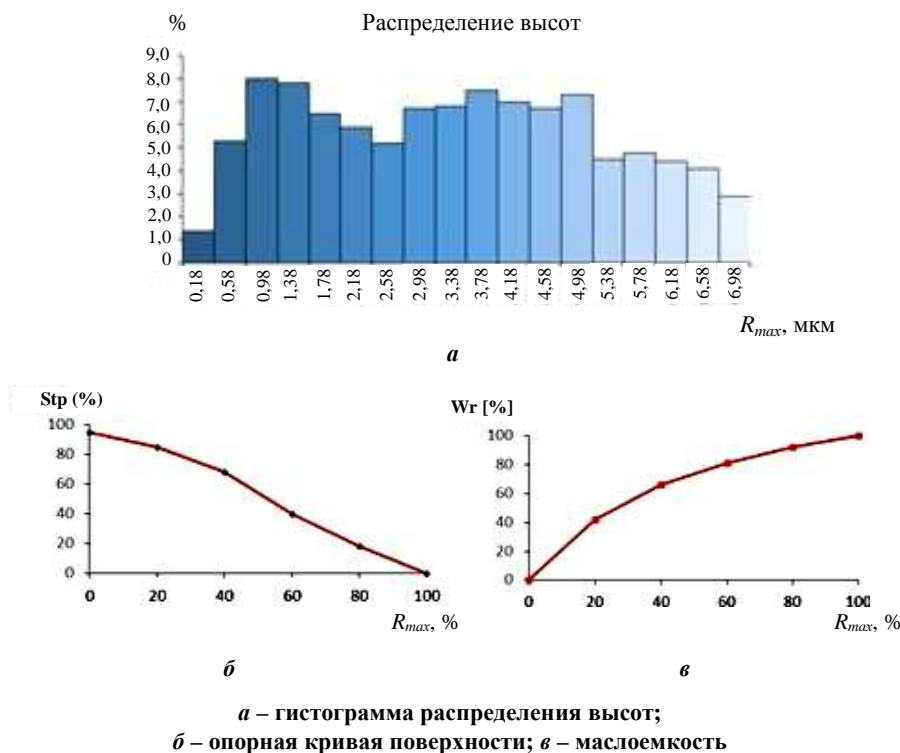
Рисунок 6. – Топографические характеристики поверхности после токарной обработки
