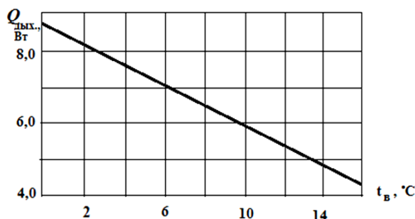
Рисунок 1. – Зависимость потерь теплоты на нагрев вдыхаемого воздуха ( Q_{дых.} ) от температуры производственной среды ( t_{в.} )
