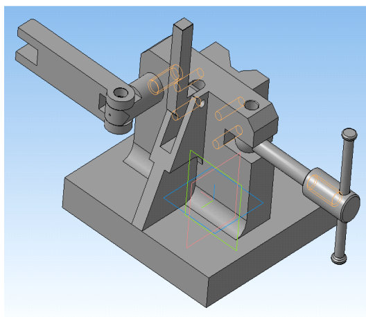
Рисунок 1. – Сборка узла
