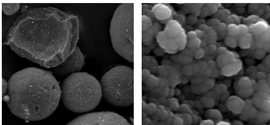
a – полые алюмооксидные микросферы; б – нанодисперсная структура поверхности
