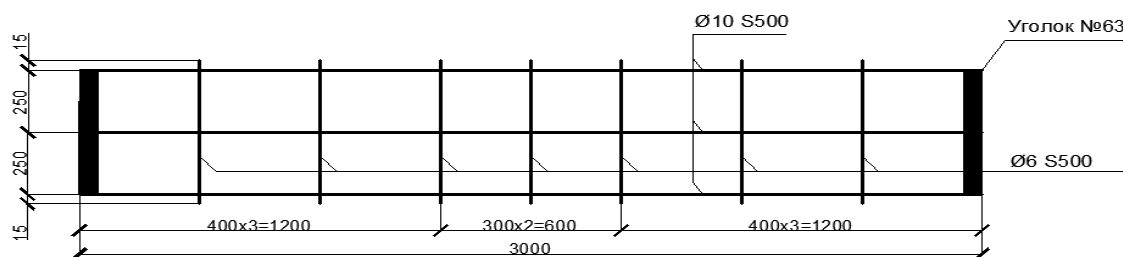
Рисунок 1. – Арматурная сетка
