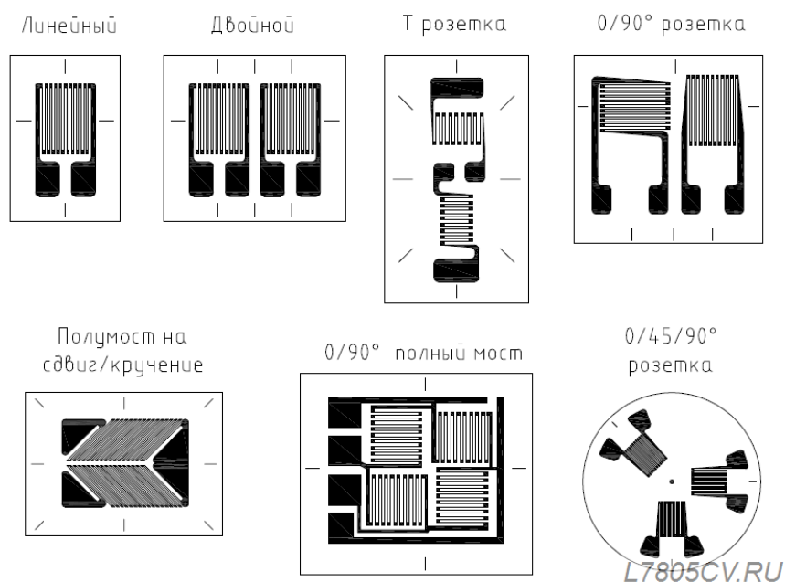
Рисунок 1. – Виды типоразмеров тензорезисторов
