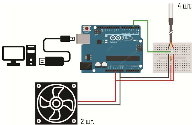
Рисунок 4. – Схема подключение датчиков температуры в “Умной стеновой панели”
