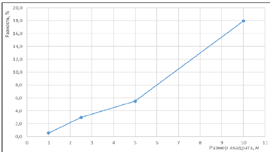
Рисунок 2. – График разности значений объема метода квадратов от метода призм
