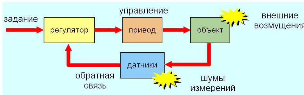
Рисунок 1. Схема системы управления
