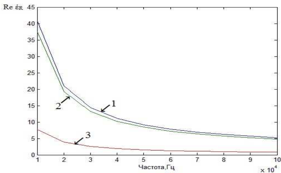
Рисунок 3. – Зависимости при F_n = 5 \cdot 10^5 Гц
